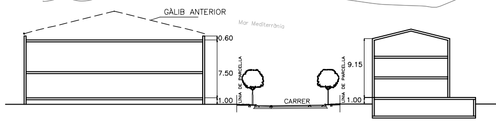
SECCIÓ TIPUS e: 1/500 (7.1/7.2a/7.2b/7.3/7.4/E.1)
